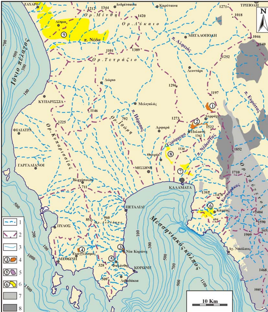
Εικ. 2. Οι θέσεις εμφάνισης των μεταλπικών σχηματισμών, που περιέχουν κροκάλες από μεταμορφωμένα πετρώματα, στη ΝΔ Πελοπόννησο. 1:υδρογραφικό δίκτυο, 2:υδροκρίτες, 3:ισοβαθείς, 4:θέσεις εμφάνισης, 5:ενότητα Μάνης, 6:ενότητα Άρνας.
