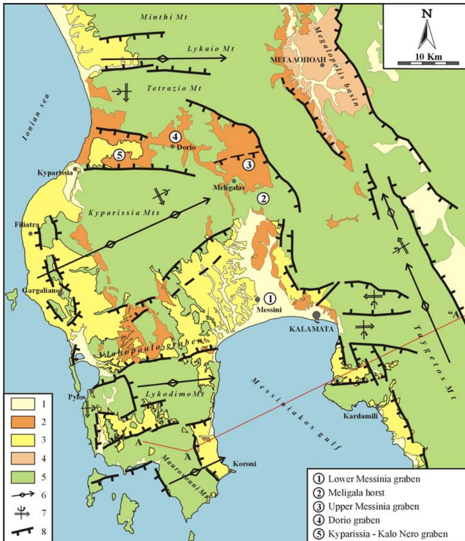
Εικ. 3.: Νεοτεκτονικές μακροδομές της ΝΔ Πελοποννήσου.
